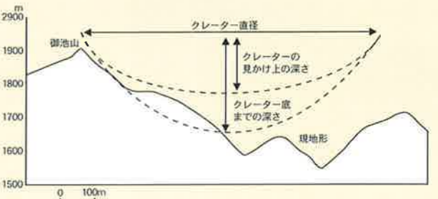
御池山隕石クレーターの断面図 Schematic cross section of the Oikeyama impact crater
